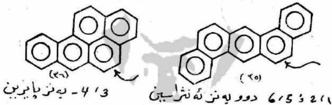
3,4 — Benzpyrene 1,2; 6,5 — Di benzanthracene
